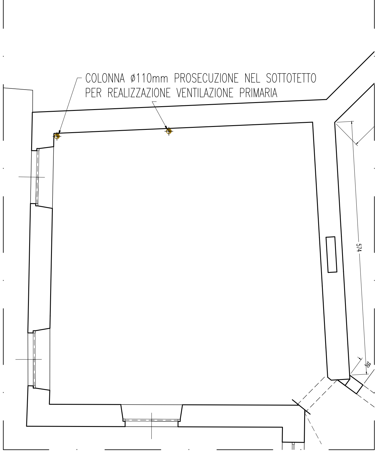
RETE FOGNATURA - PIANO PRIMO
