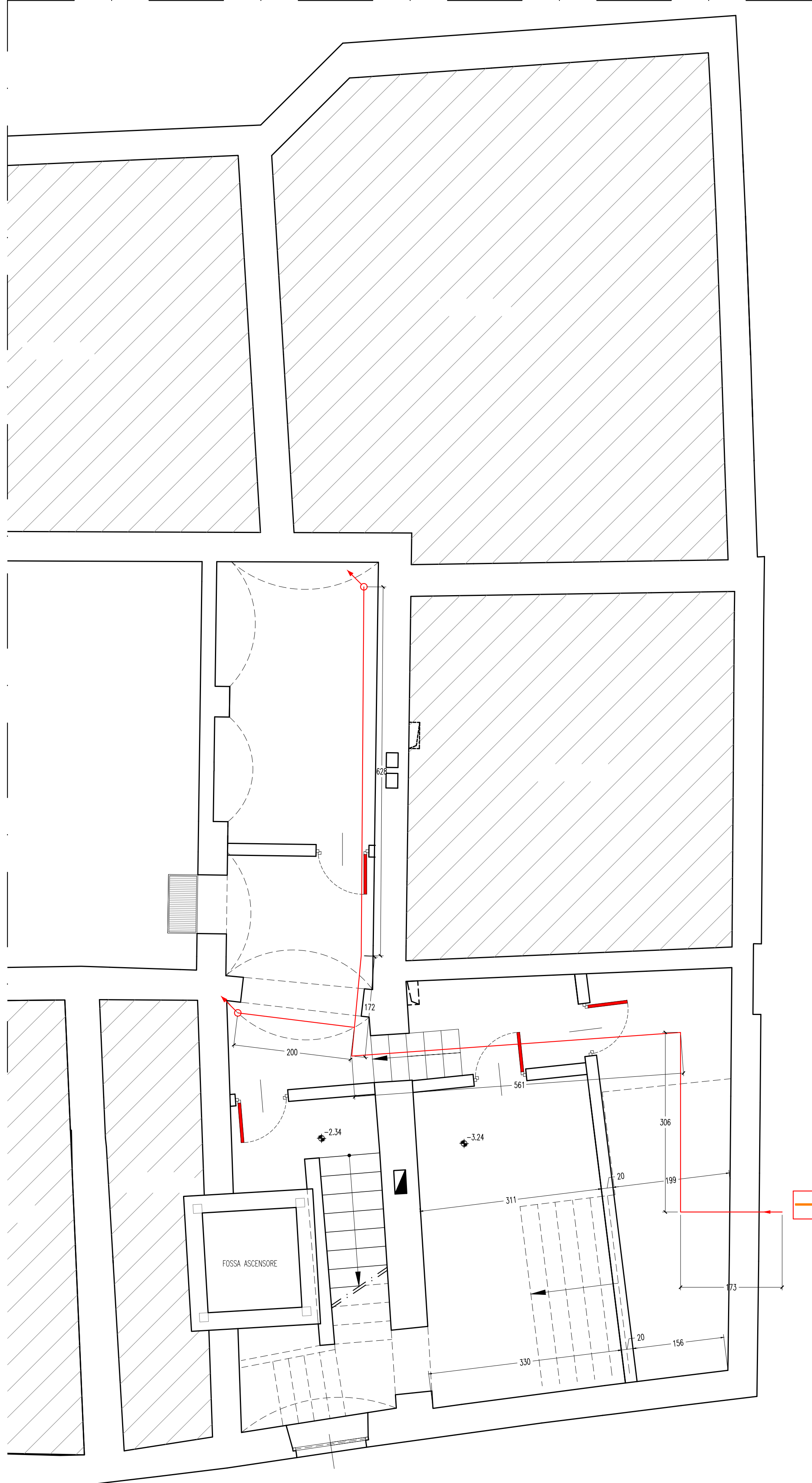
PIANTA PIANO INTERRATO
